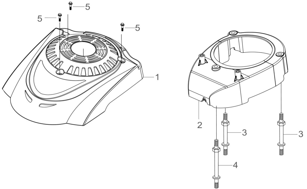
FIG.7 SHIELD, FAN (E07)
