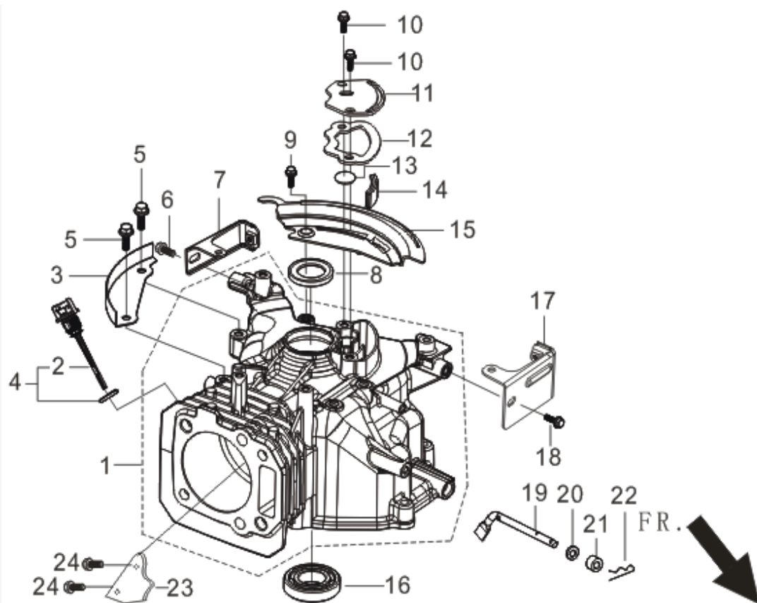
FIG.1 CRANKCASE. (E01)
