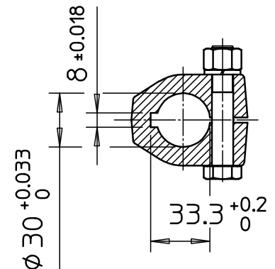
Sez. A:A
